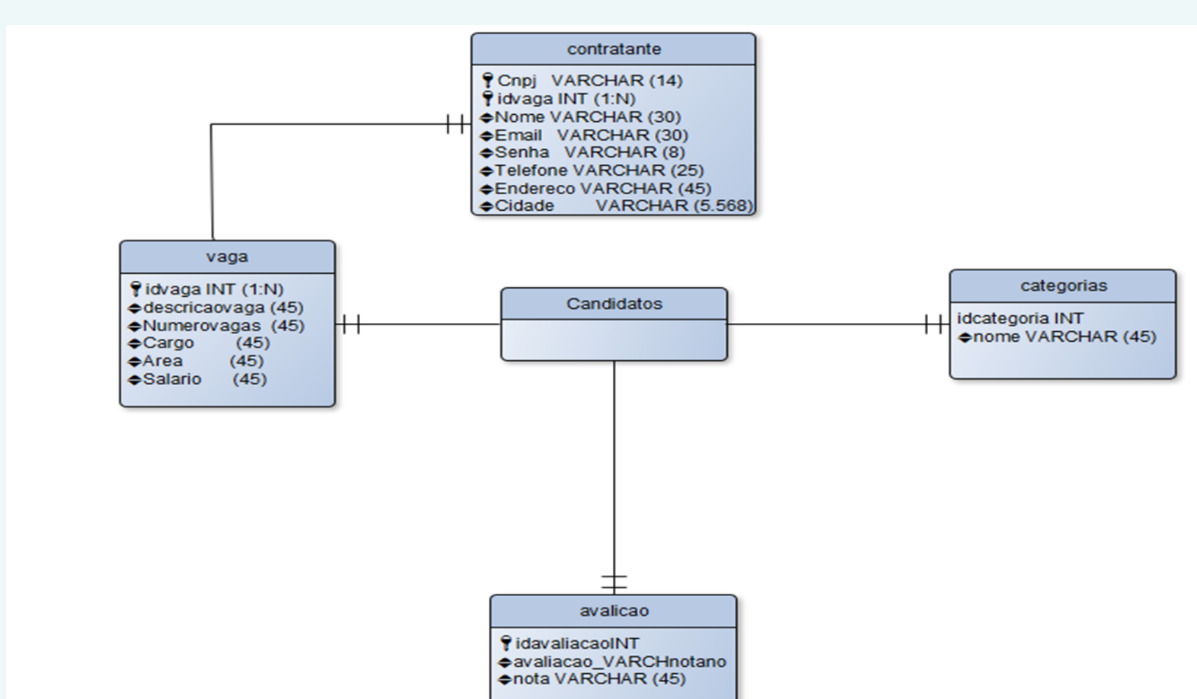
Figura 2. Modelo de dados
